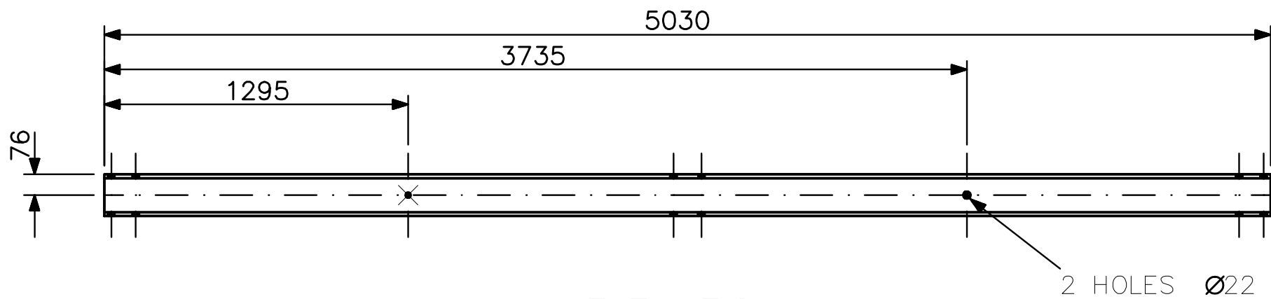
ELEVATION
